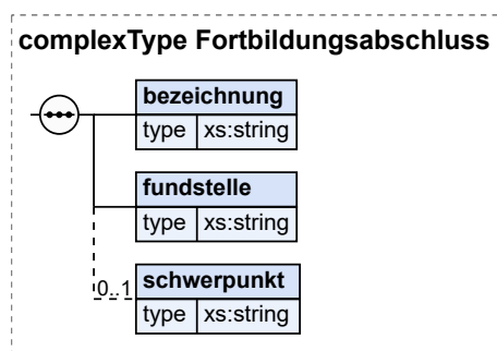
Abbildung II.6.6. Fortbildungsabschluss
