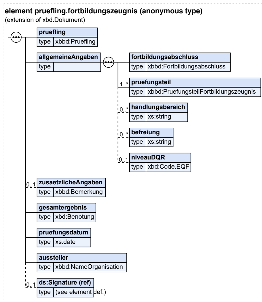
Abbildung II.7.2. pruefling.fortbildungszeugnis.0002
