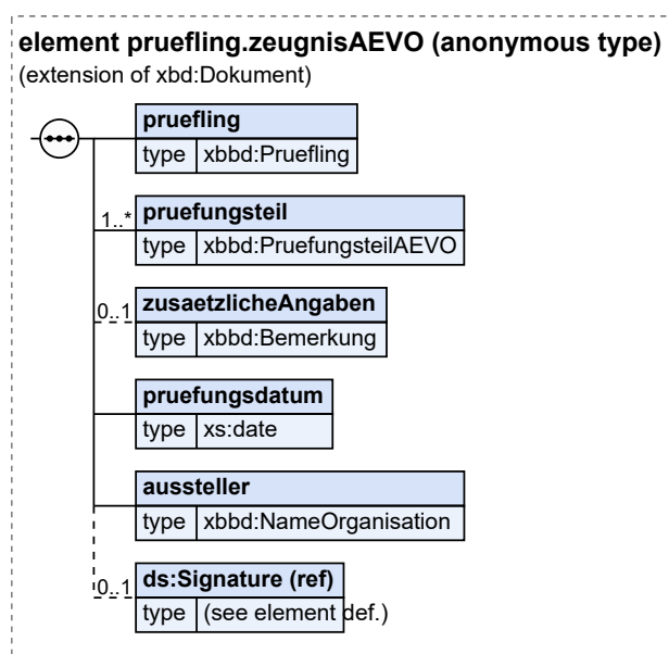
Abbildung II.7.3. pruefling.zeugnisAEVO.0003
