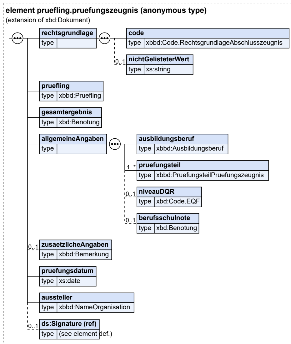
Abbildung II.7.1. pruefling.pruefungszeugnis-0001
