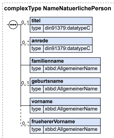
Abbildung II.5.8. NameNatuerlichePerson
