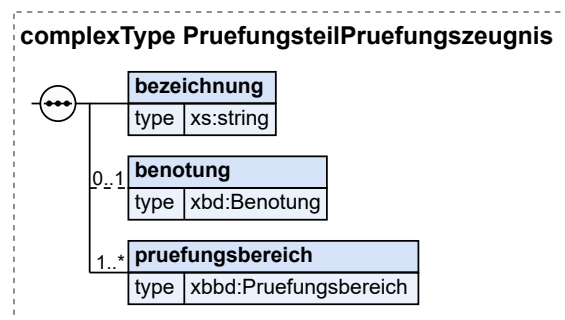
Abbildung II.6.12. PruefungsteilPruefungszeugnis
