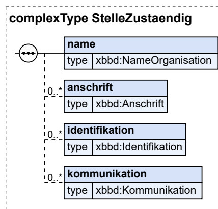
Abbildung II.5.12. StelleAusstellendStelleZustaendig
